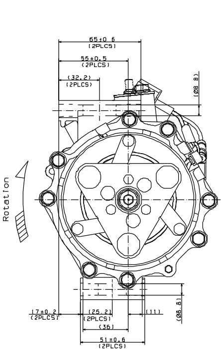
SECT DD
