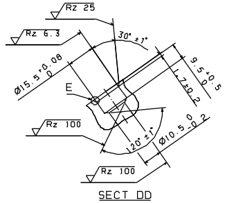
SECT DD
